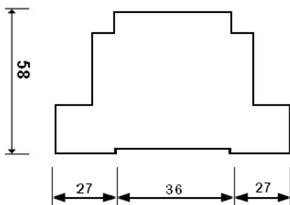
VISTA DI LATO
